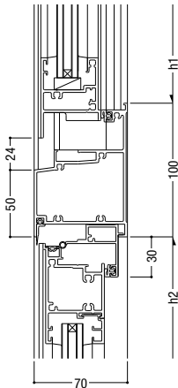
33 FIX / 外開き・たてすべり出し
