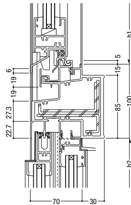
23 外開き / 外開き たてすべり出し / たてすべり出し
