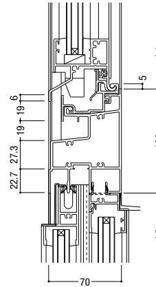
19 内倒し排煙 / 両袖可動・中央可動・中央引き分け
