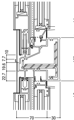
21 インベイ内倒し排煙 / 両袖可動・中央可動・中央引き分け
