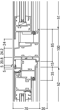
34 FIX / 外開き・たてすべり出し
