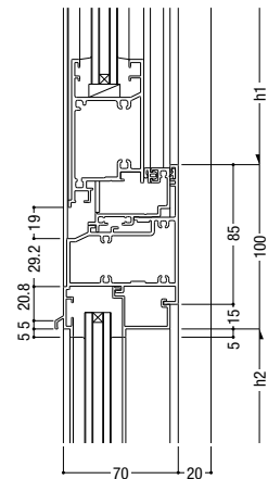
72 外倒し排煙(インペイと共通) / FIX
