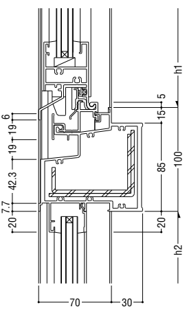
82 内倒し排煙 / FIX
