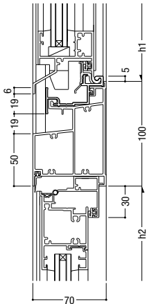
35 外倒し排煙(インペイと共通) / 内開き
