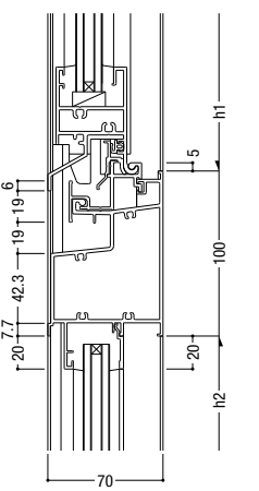
81 内倒し排煙 / FIX
