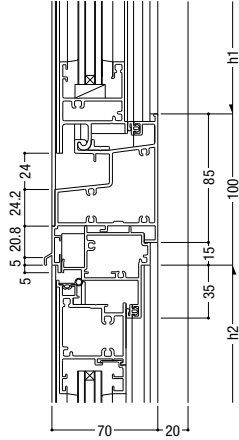
30 突出し排煙 / 外開き・たてすべり出し
