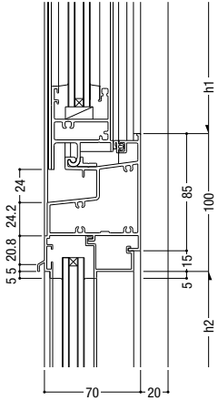
80 内倒し排煙 / FIX
