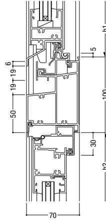
31 インペイ内倒し排煙 / 外開き・たてすべり出し
