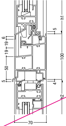
53 インペイ内倒し排煙 / たて軸回転
