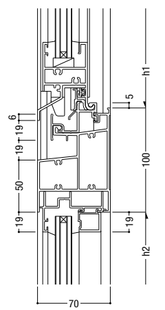
84 突出し排煙 / FIX
