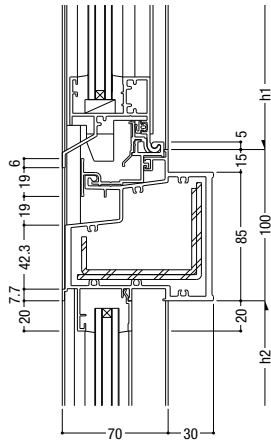
94 インペイ内倒し排煙 / FIX
