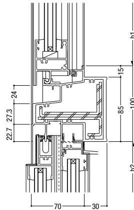
22 FIX / 両袖可動・中央可動・中央引き分け
