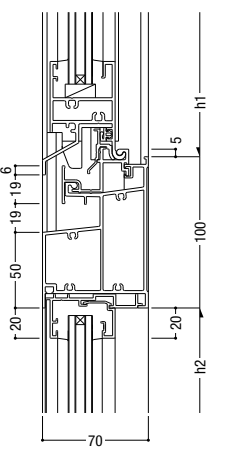
83 突出し排煙 / FIX
