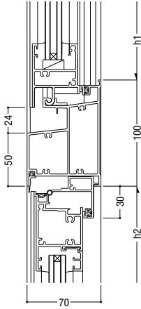
29 突出し排煙 / 外開き・たてすべり出し
