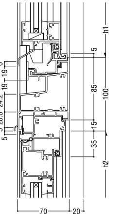
36 外倒し排煙(インペイと共通) / 内開き
