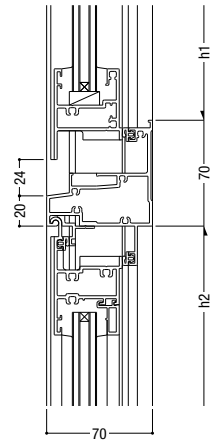
59 外倒し排煙(インペイと共通) / 片開きドア・両開きドア
