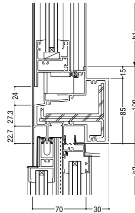
24 外開き / 外開き たてすべり出し / たてすべり出し
