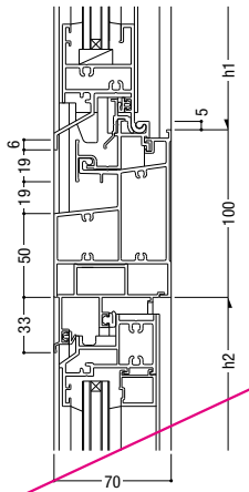
41 インベイ内倒し排煙 / 内開き
