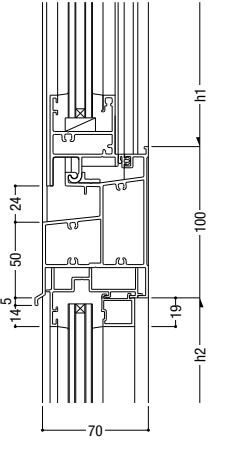
79 内倒し排煙 / FIX
