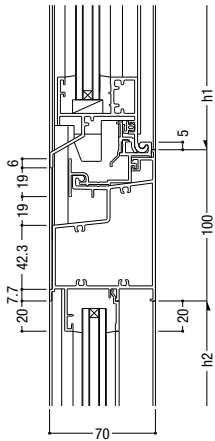
93 インペイ内倒し排煙 / FIX
